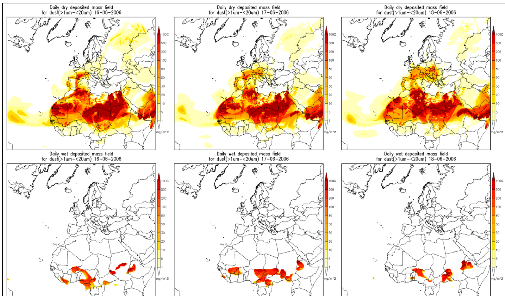
Fig. 19 – – Mappe della deposizione media giornaliera di polvere minerale (in mg/m 2 ) con diametro aerodinamico compreso tra 1 e 20 µm, dal 16 al 18 giugno; deposizione secca (sopra), deposizione umida (sotto).
