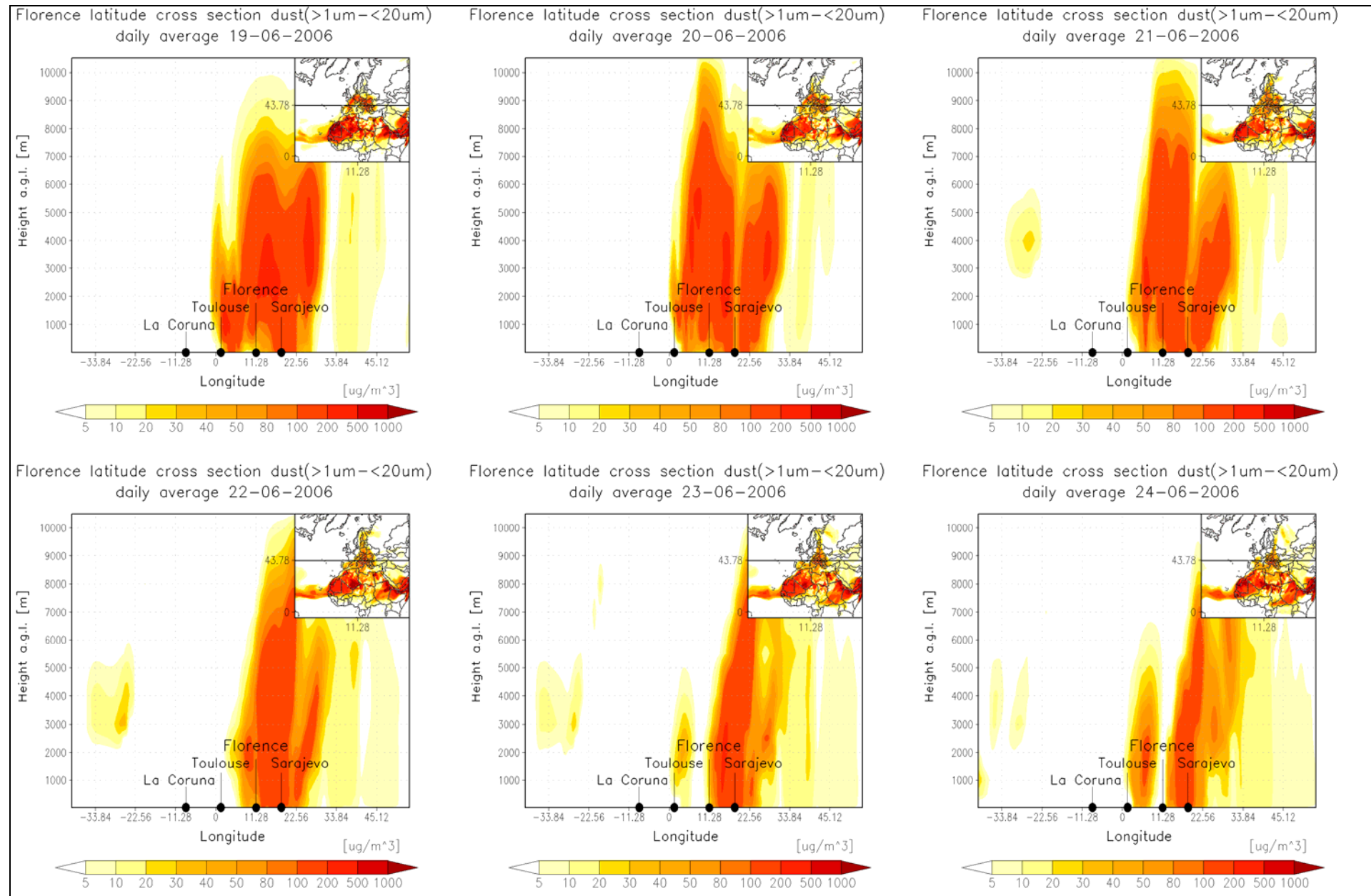
Fig. 20 – Sezione verticale (10 – 10500 m) della concentrazione media giornaliera della somma di CCR1 e CCR2, alla latitudine di Firenze, ( \mu\text{g}/\text{m}^3 ), dal 19 al 24 giugno.
